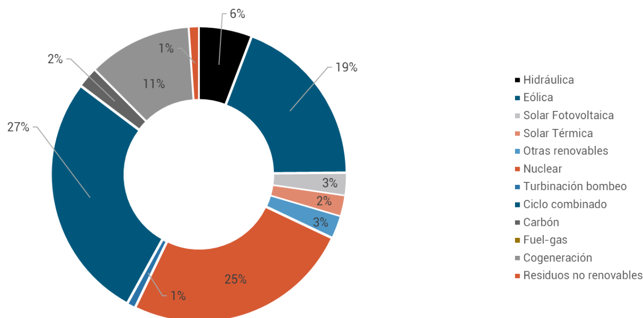
GENERACIÓN TIPO PRODUCCIÓN (MWh) SEPTIEMBRE 2019
